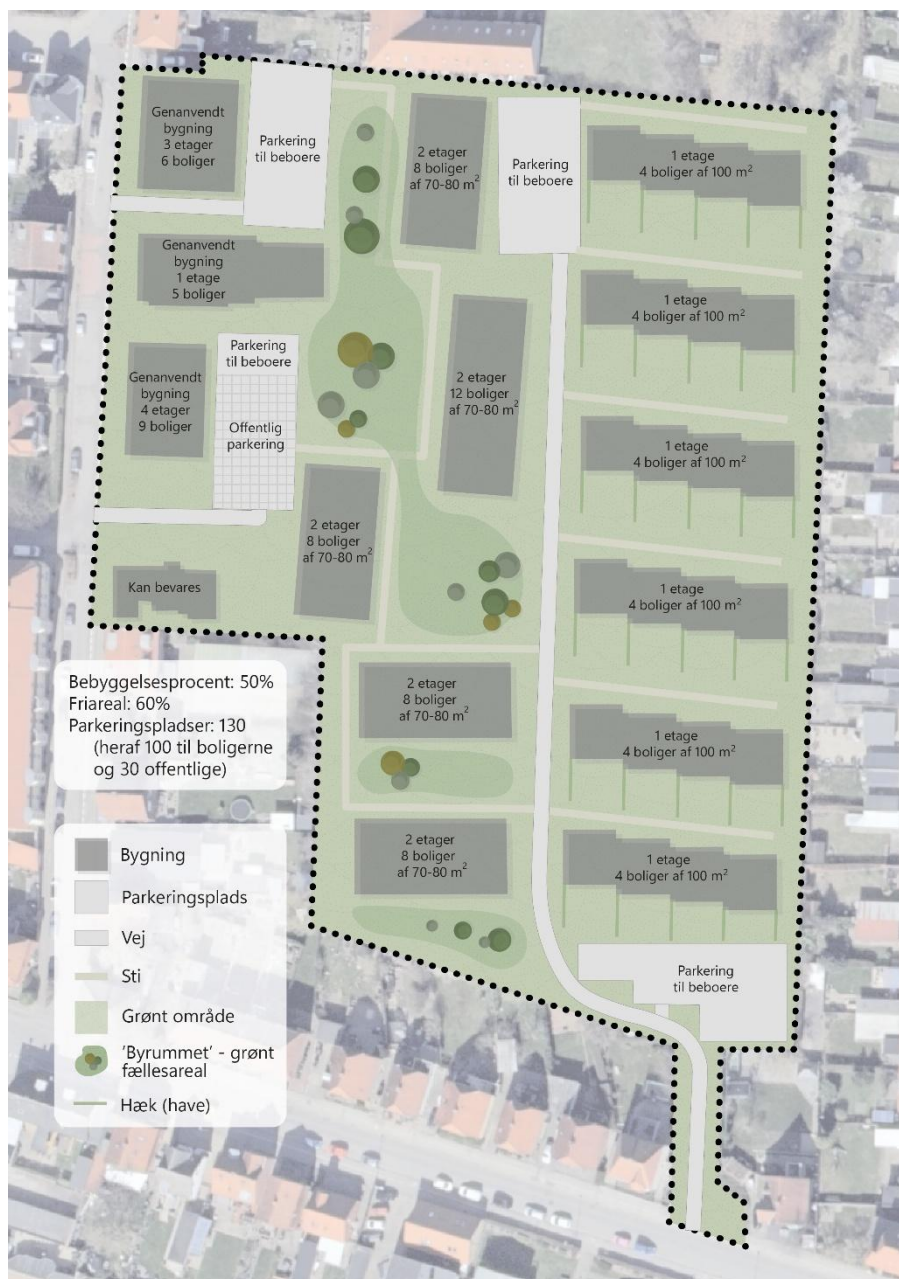
Figur 14. Planskitse, eksempel 1
